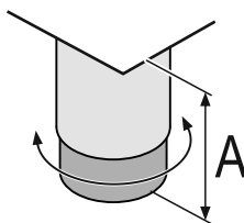
Fig. 9 Nastaviteľná noha sa dá prestaviť od A = 115 \text{ mm} ( 4 \frac{1}{2} \text{ in} ) do 175 \text{ mm} ( 6 \frac{7}{8} \text{ in} ).
